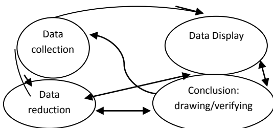
Komponen dalam analisis data ( interactive model )
